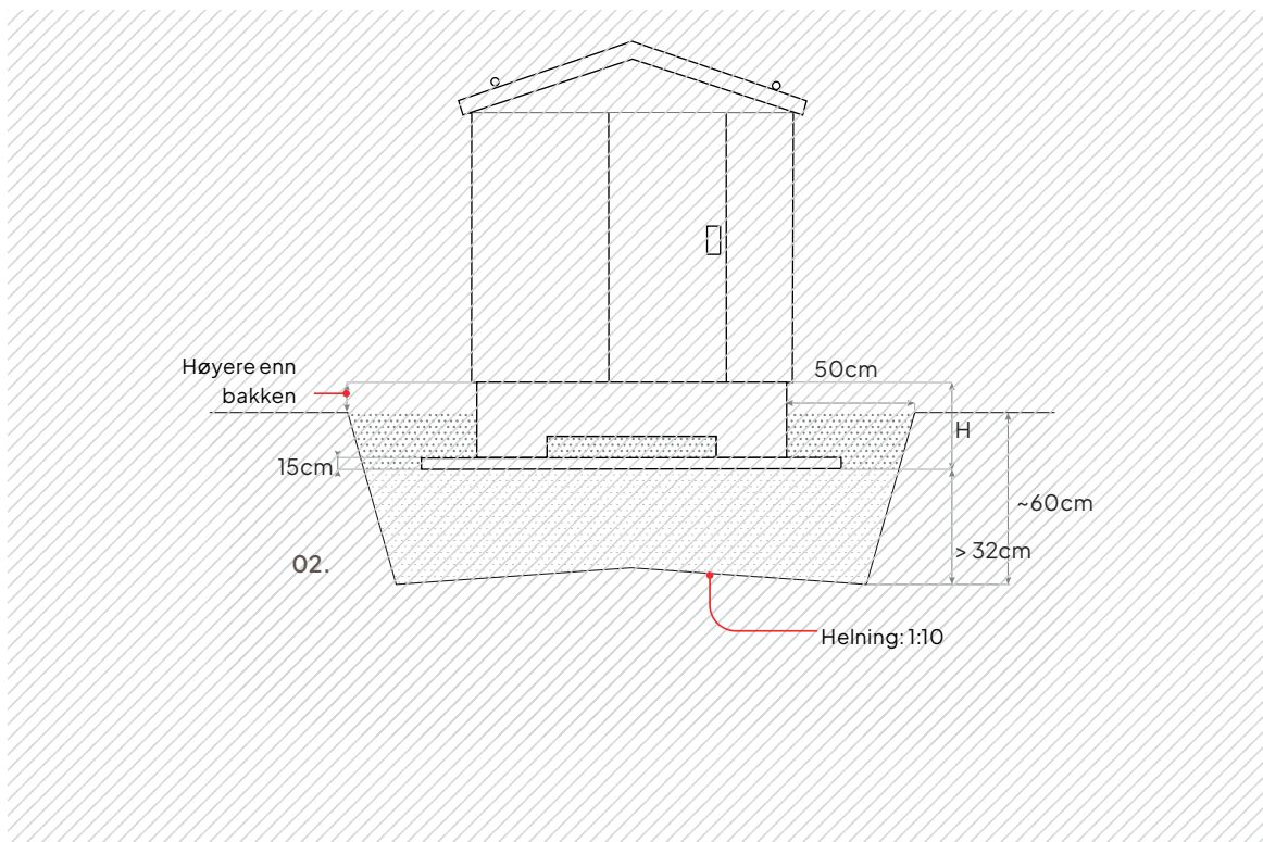
01. Fundamentgrop for de fleste tilfeller.
